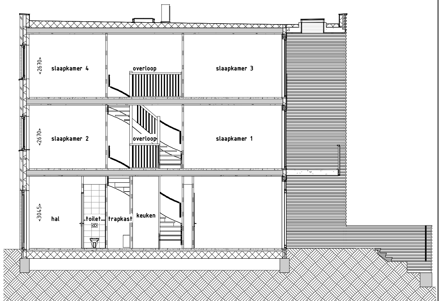
Doorsnede:
