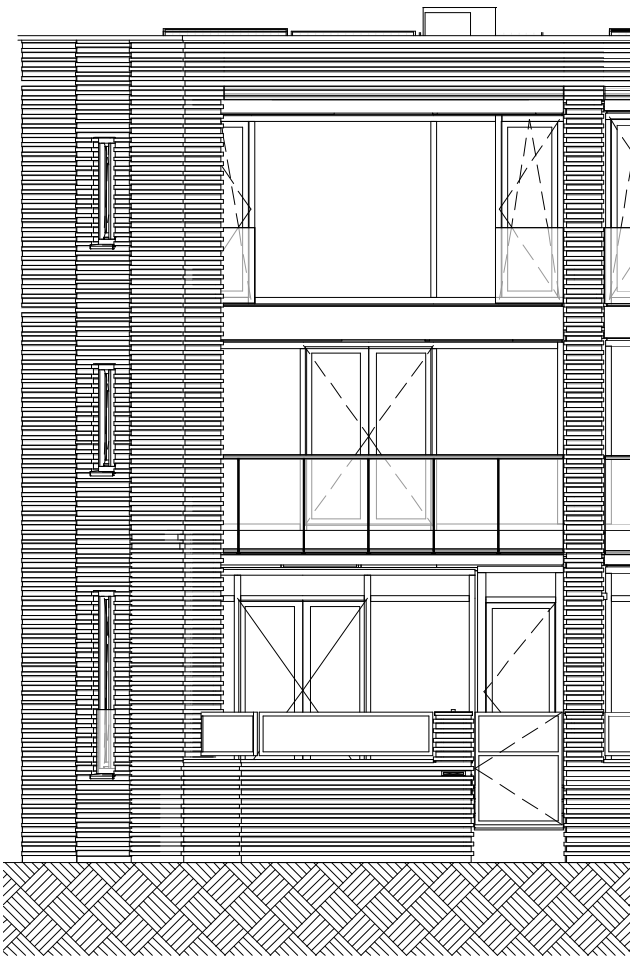
Voorgevel:
