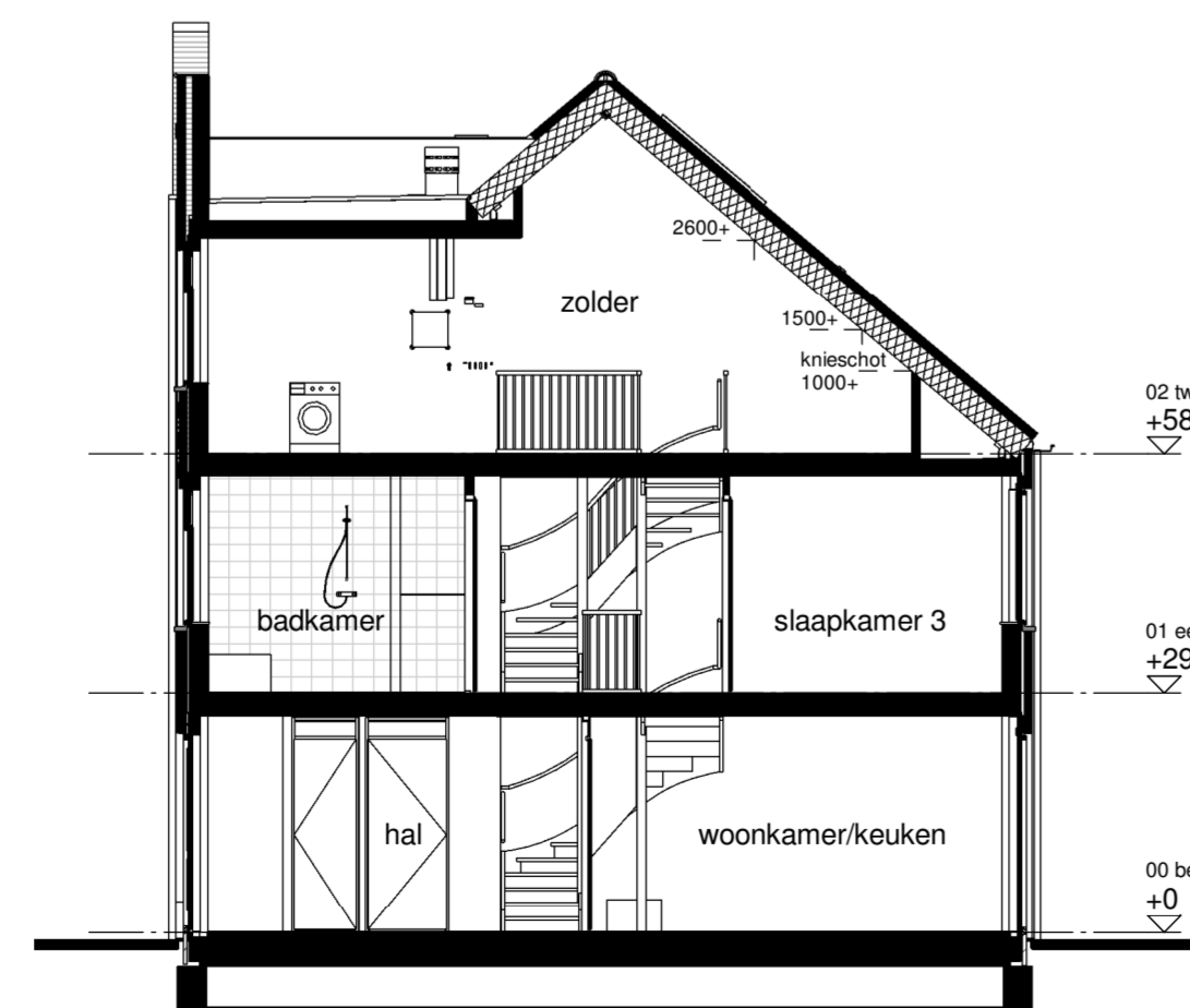
Doorsnede C2
