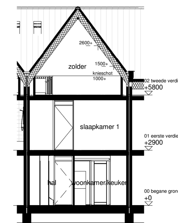
Doorsnede C3a
