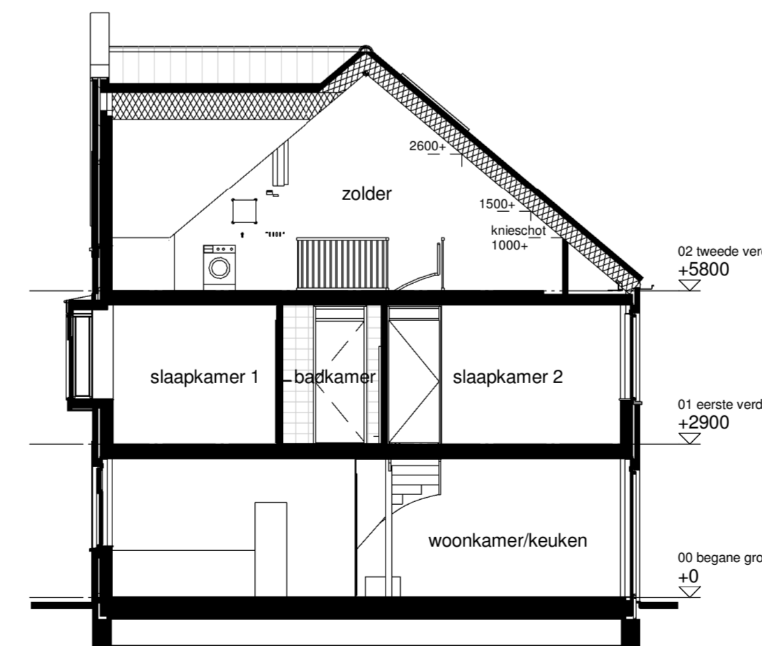
Doorsnede C3
