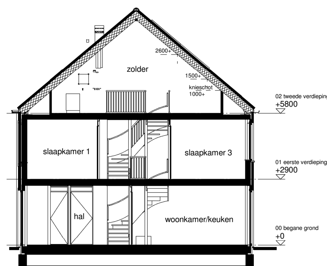
Doorsnede C1
