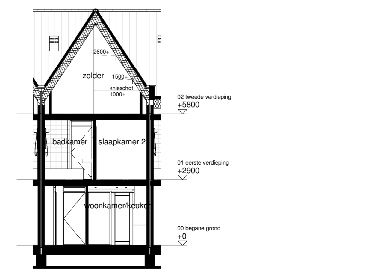
Doorsnede D3a
