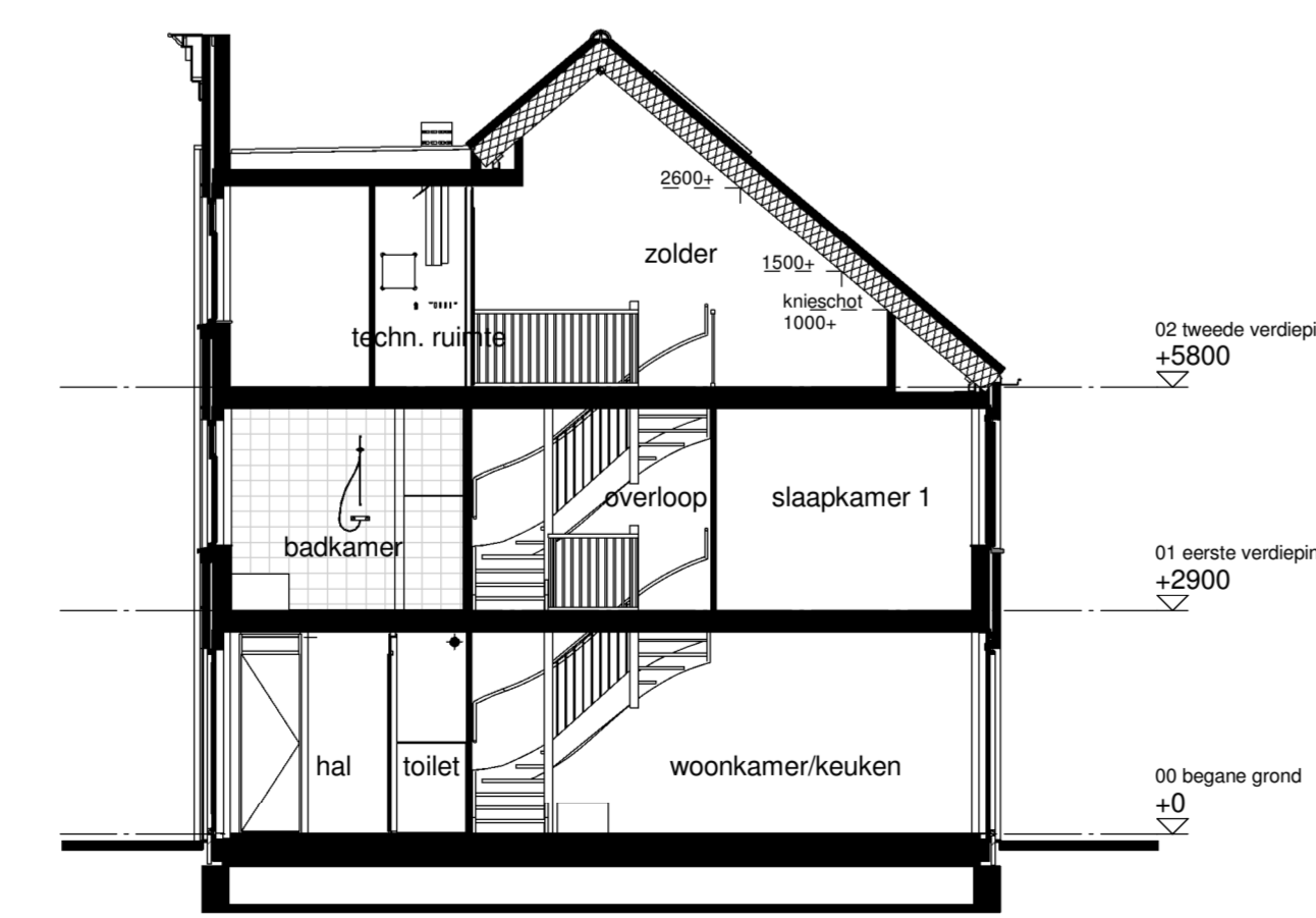
Doorsnede D2
