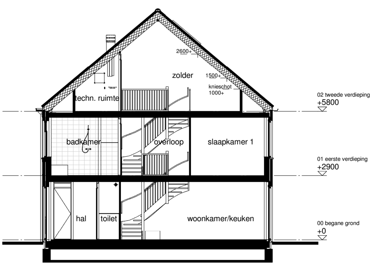
Doorsnede D1
