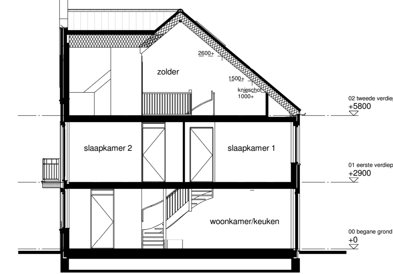
Doorsnede D3
