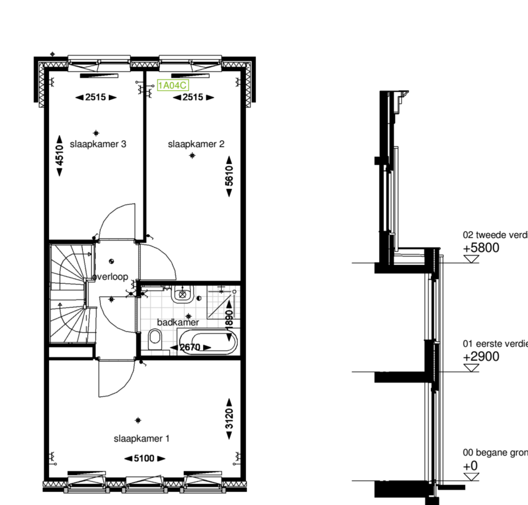
Optie C13.1: Principe trapkast bnr: 56 t/m 65, 79 t/m 88
