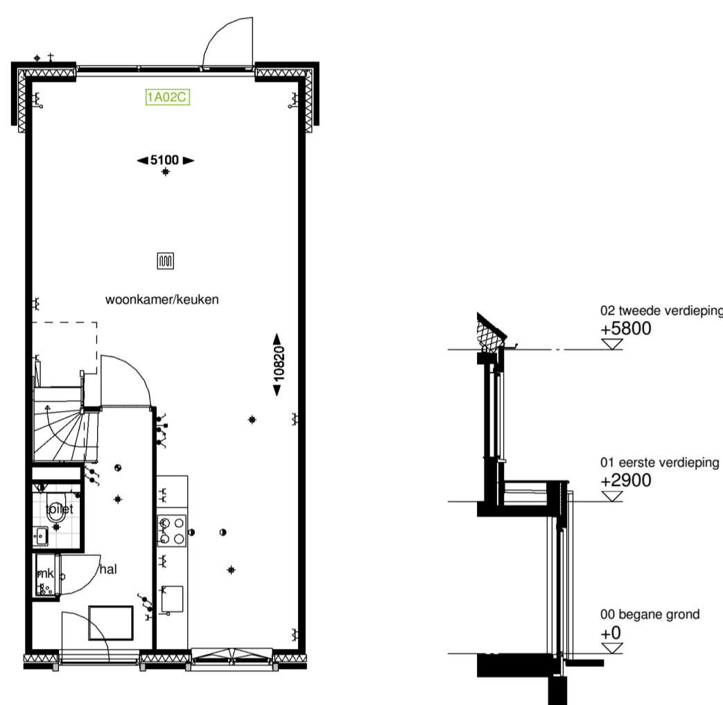
Optie C5.1: Principe dakkapel op de voorgevel bnr: 56, 58, 60, 61, 64, 86, 87
