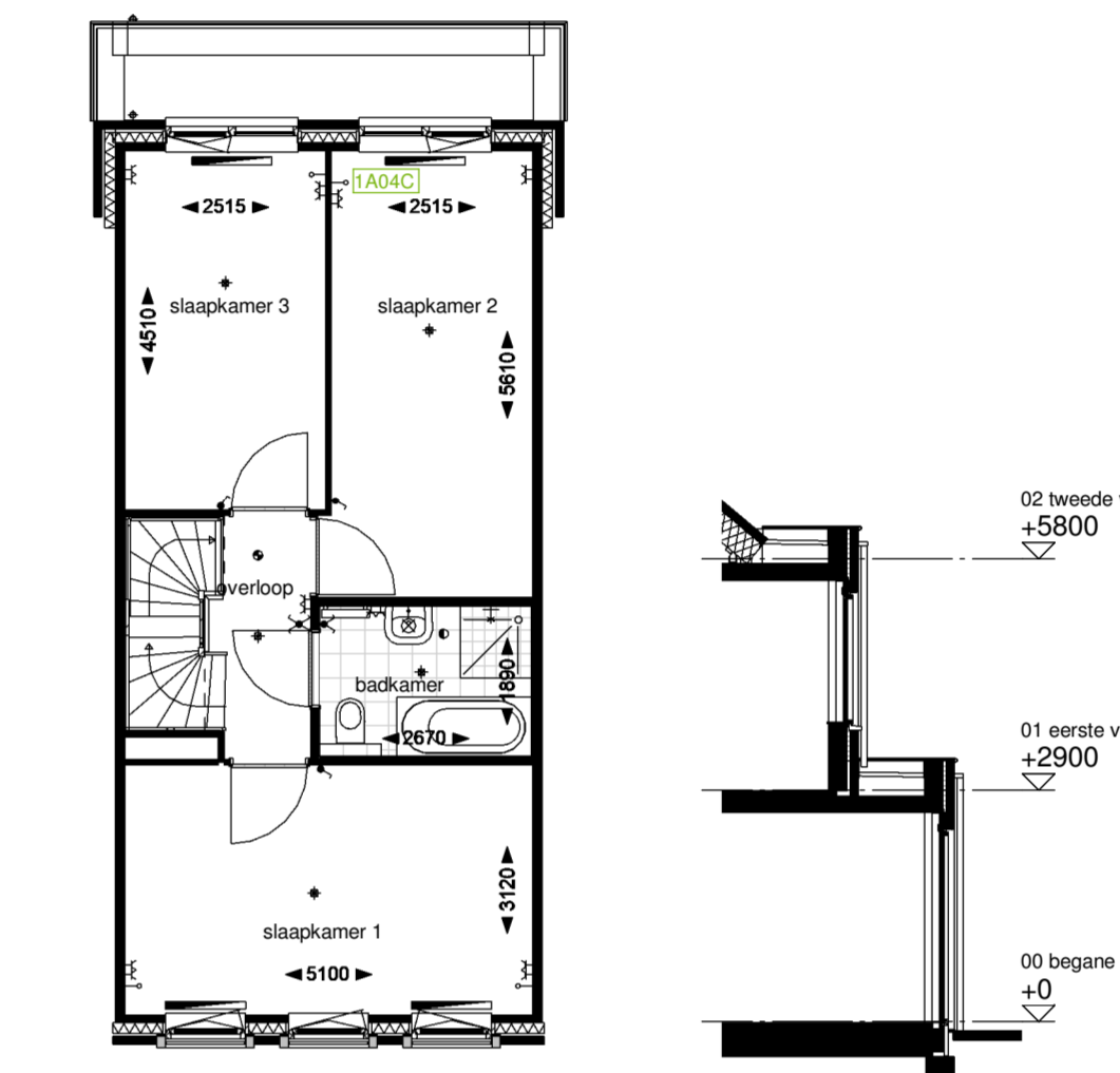
Optie C10.1: Principe indeling midden badkamer met apart toilet (alleen i.c.m. optie C3.1 / C3.2 en C13.1) bnr: 56 t/m 65, 79 t/m 88
