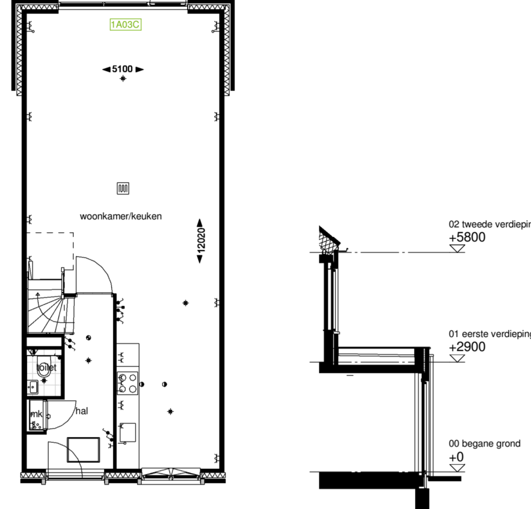
Optie C7.1: Principe dakraam voorgevel afmeting 1,34 x 1,40m bnr: 56, 58, 60, 61, 64, 86, 87
