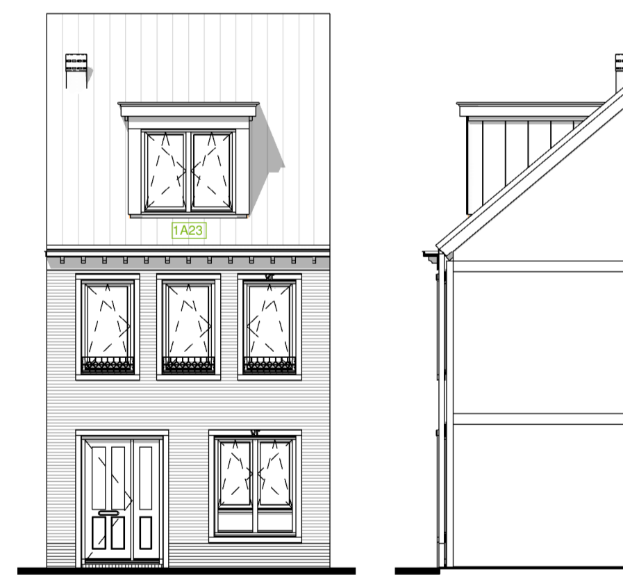
Optie C5.1: Principe dakkapel op de voorgevel bnr: 56, 58, 60, 61, 64, 86, 87
