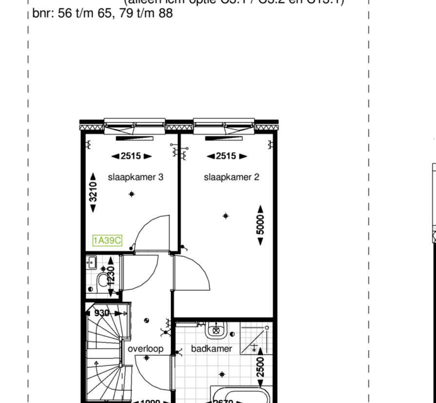
Optie C9.1: Principe indeling midden badkamer bnr: 57, 58, 59, 60, 79
