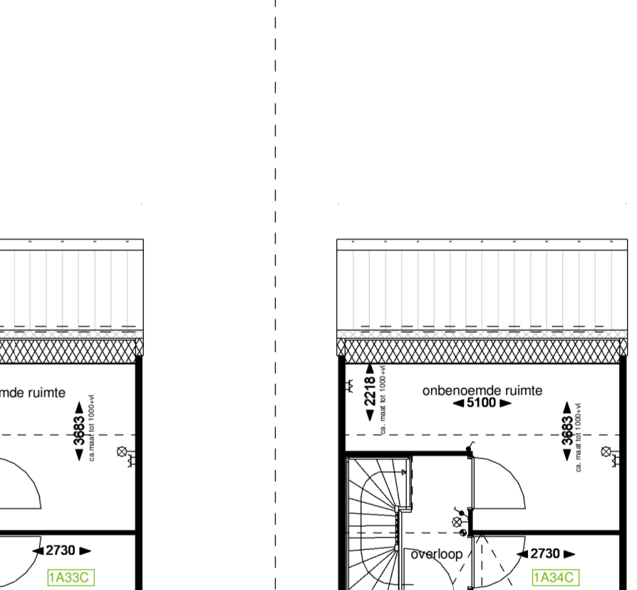
Optie C11.3: Principe zolderindeling bnr: 79, 80, 85, 88
