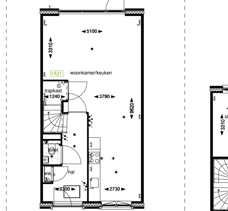
Optie C15.1: Principe schuifpui bnr: 56 t/m 65, 79 t/m 88
