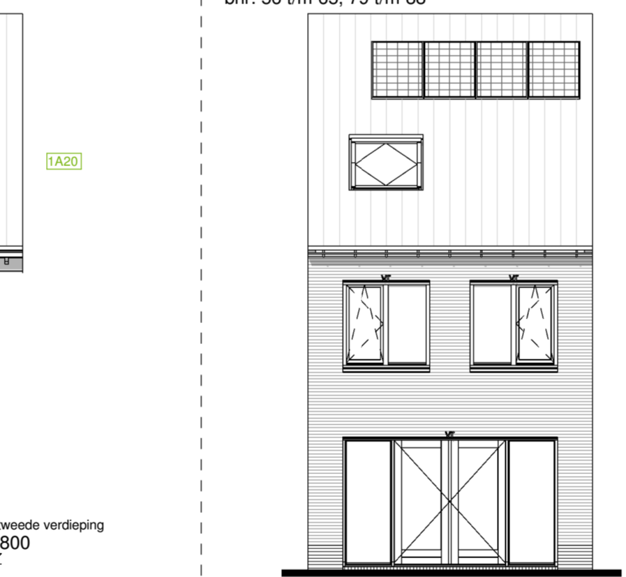
Optie C8.1: Principe dakraam achtergevel afmeting 1,34 x 1,40m bnr: 56 t/m 64, 79 t/m 88
