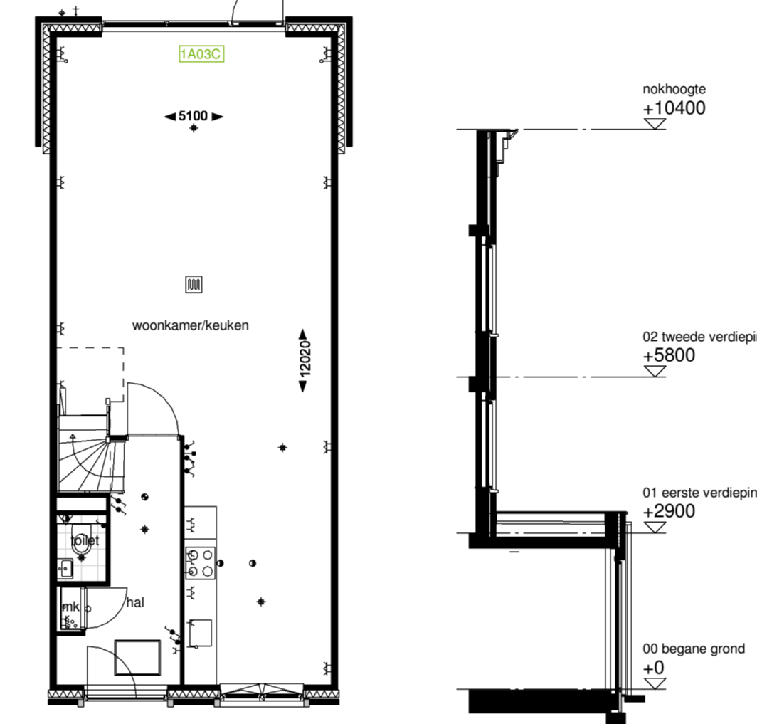
Optie C8.1: Principe dakraam achtergevel afmeting 1,34 x 1,40m bnr: 56 t/m 64, 79 t/m 88
