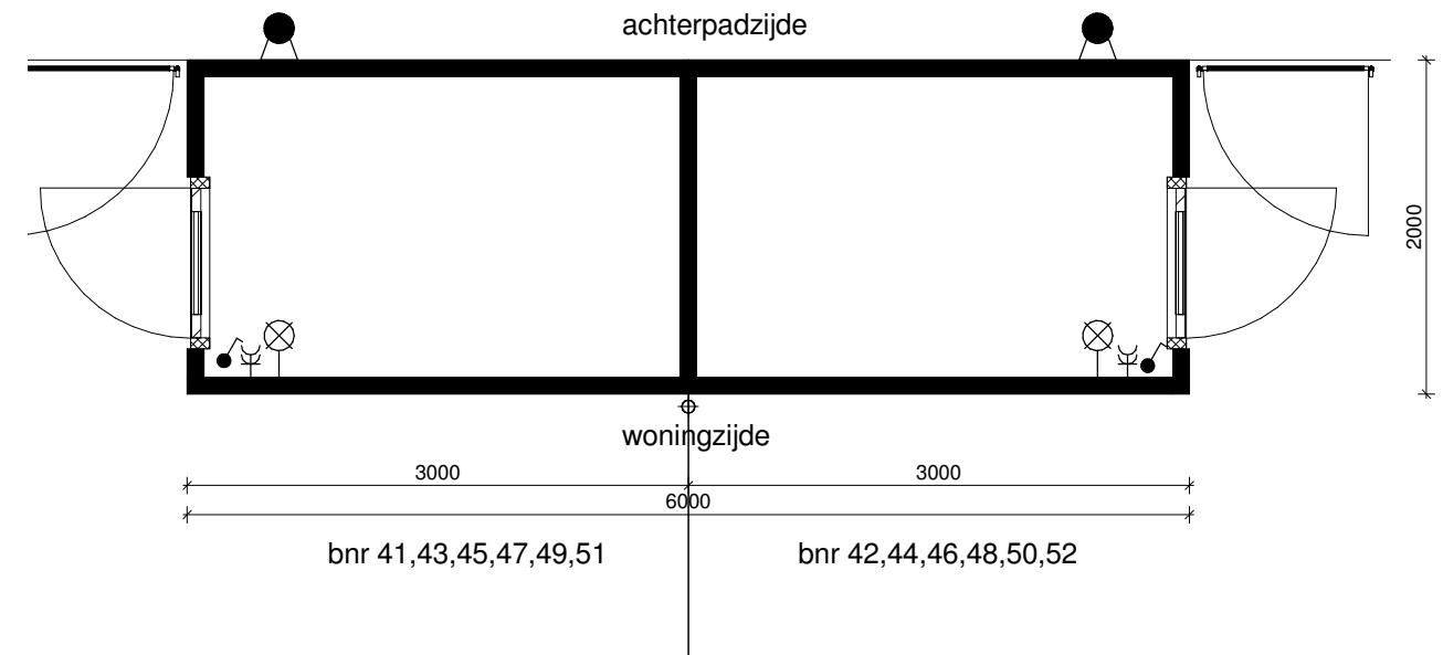
Plattegrond 1 : 50
