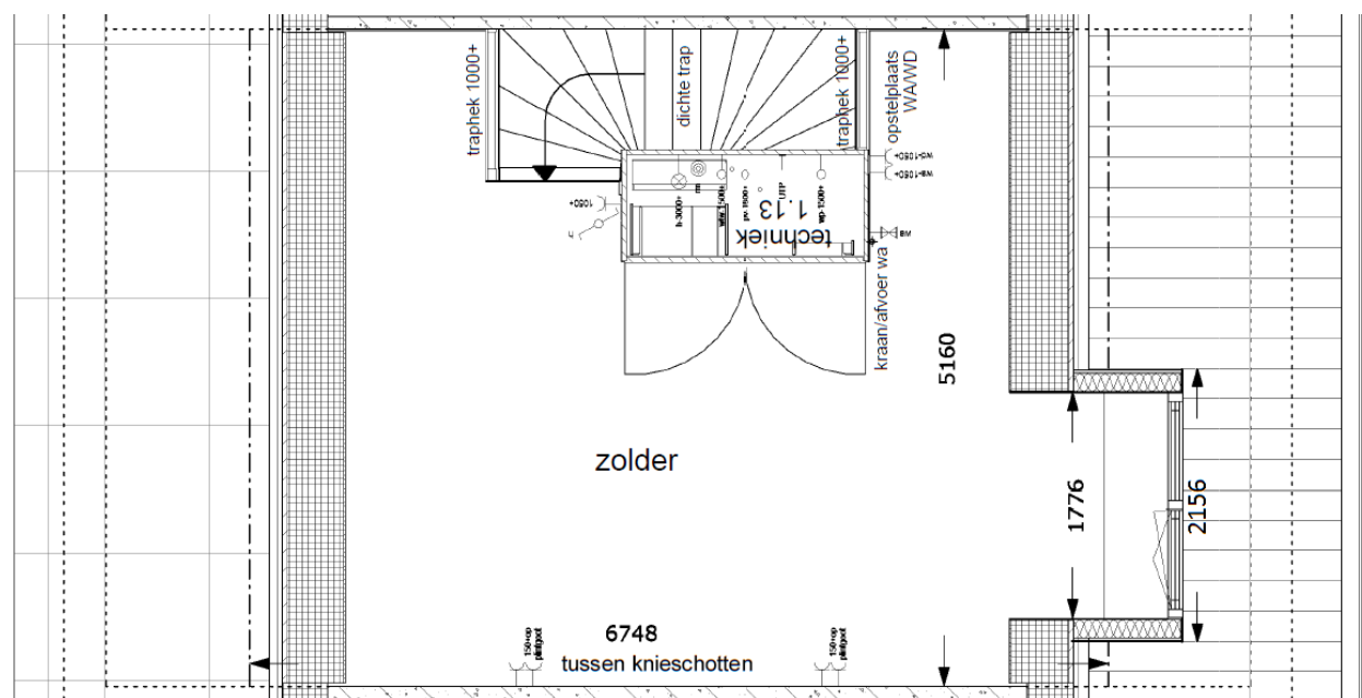
Voorbeeld plattegrond zolderverdieping met dakkapel
