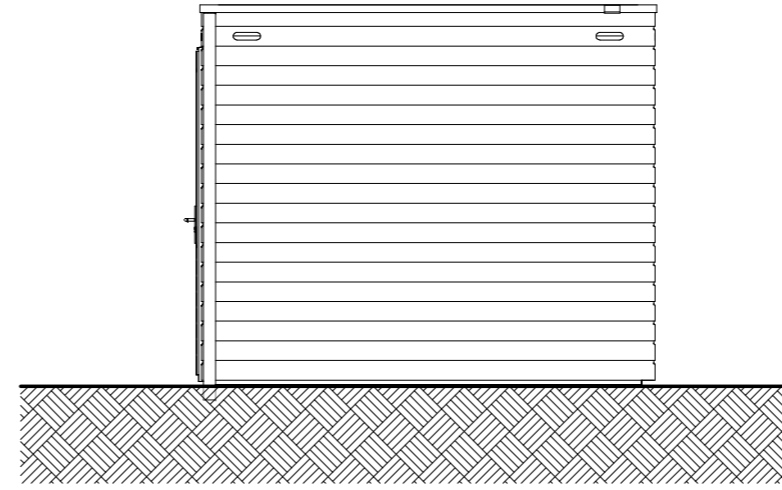
zijgevel rechterberging 1 : 50
