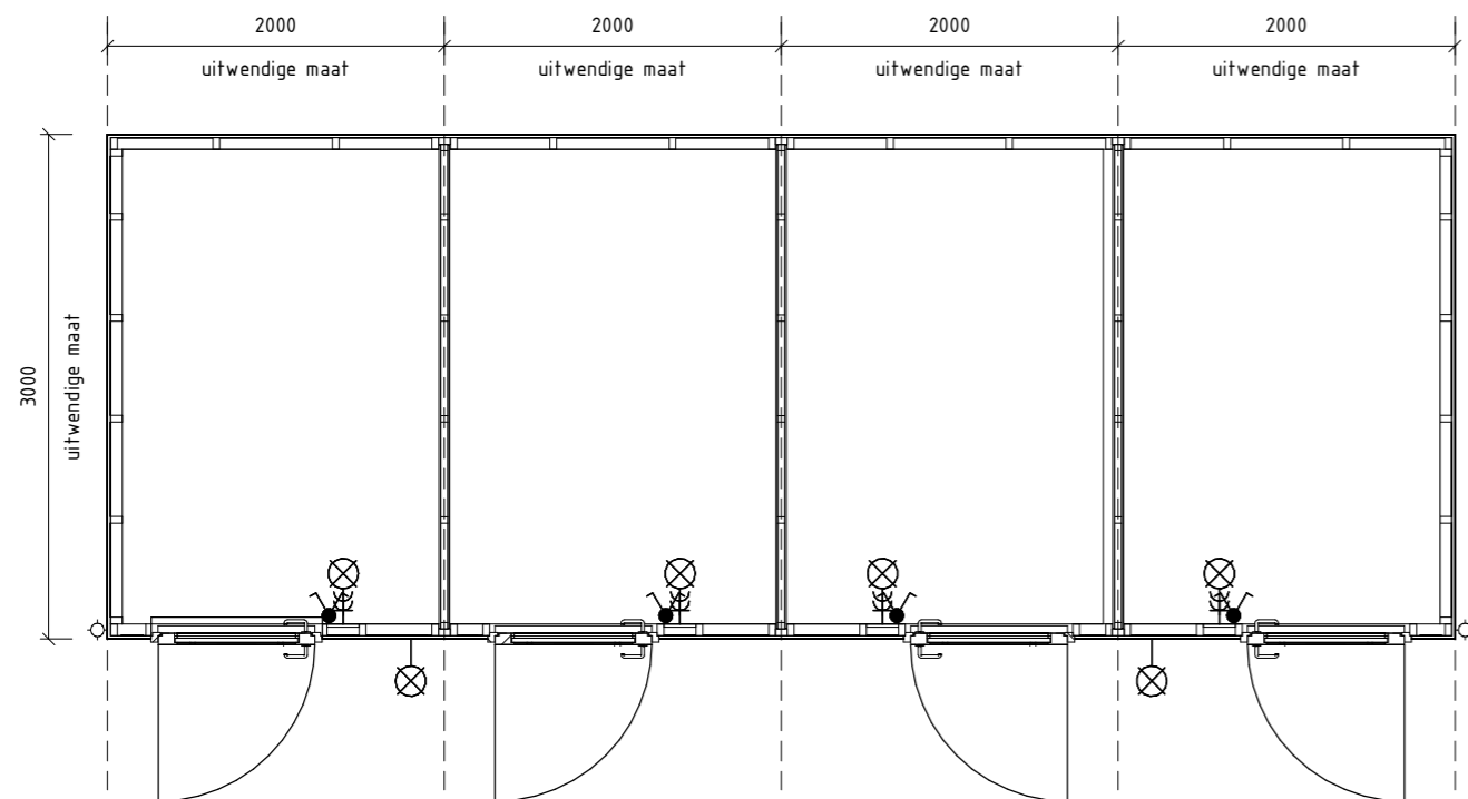
000 4 serie 1 : 50
