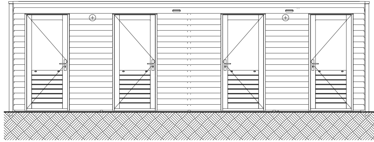
gevel binnentereinzijde 1 : 50
