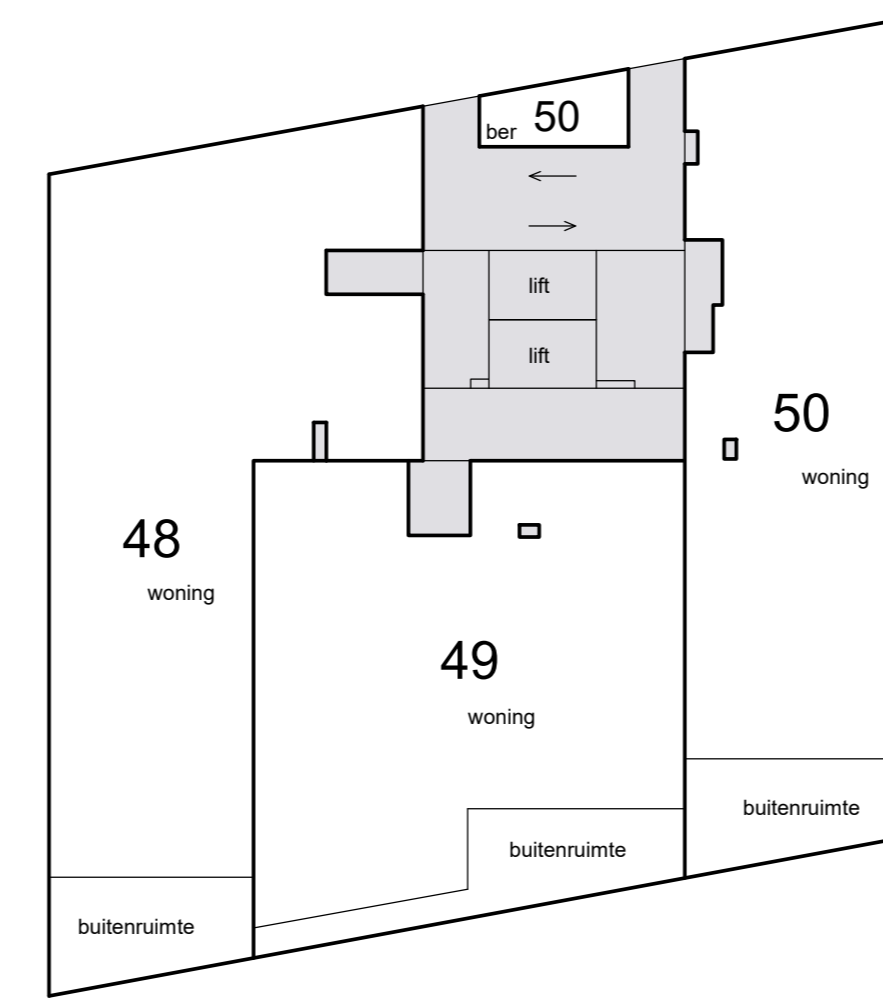
16e etage
