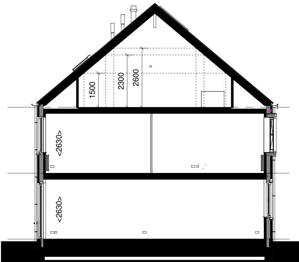
Doorsnede 1 : 100
