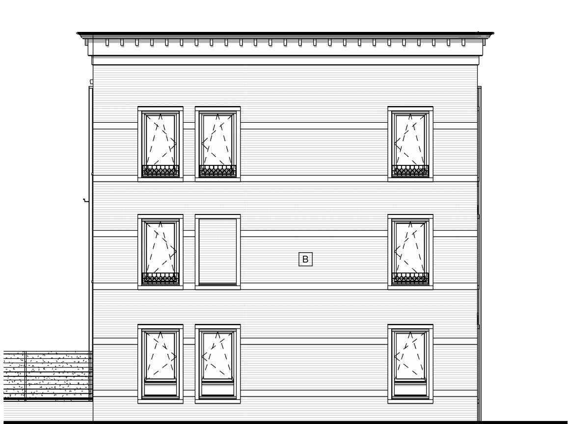
Linker zijgevel
