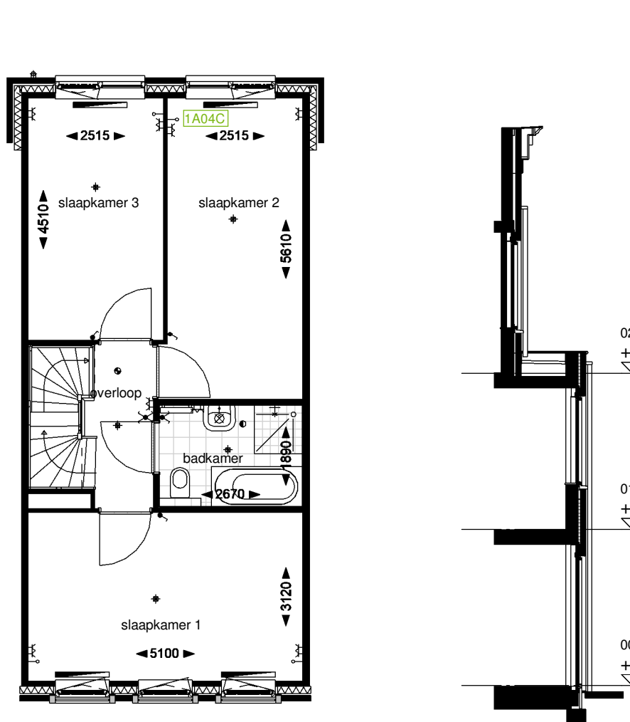
Optie C9.1: Principe indeling midden badkamer bnr: 57, 58, 59, 60, 79, 94 t/m 96
