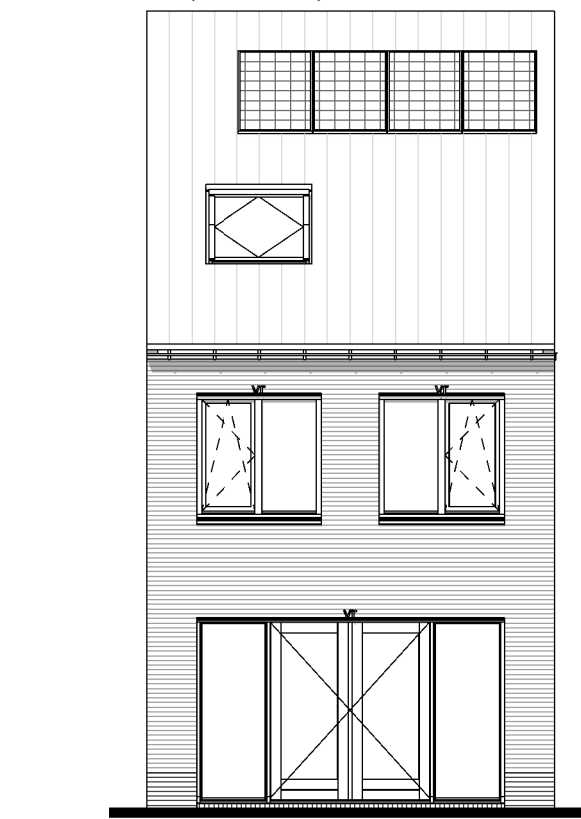
Optie C12.1: Principe grote pui met dubbele deuren achtergevel bnr: 56 t/m 65, 79 t/m 88, 89 t/m 101
