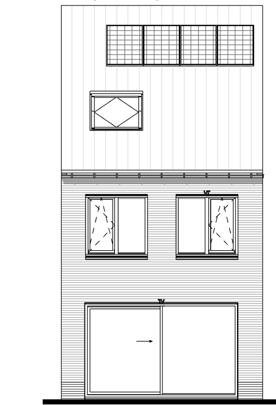
Optie C15.1: Principe schuipui bnr: 56 t/m 65, 79 t/m 88, 89 t/m 101
