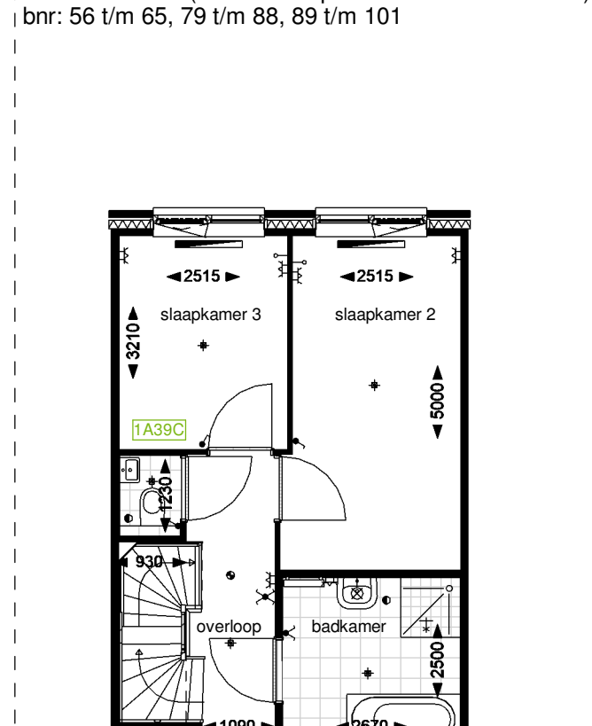
Optie C10.1: Principe indeling midden badkamer met apart toilet (alleen iem optie C3.1 / C3.2 en C13.1) bnr: 56 t/m 65, 79 t/m 88, 89 t/m 101
