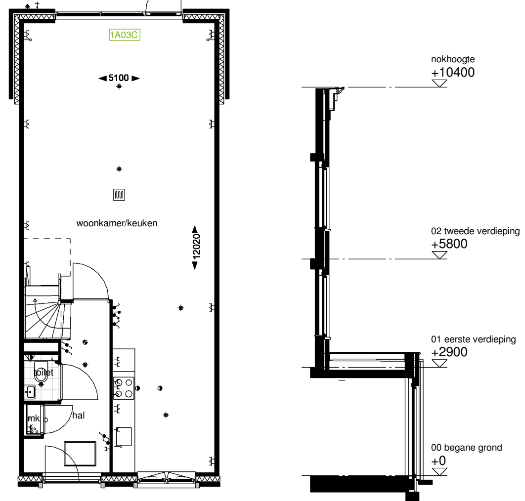
Optie C12.1: Principe grote pui met dubbele deuren achtergevel bnr: 56 t/m 65, 79 t/m 88, 89 t/m 101
