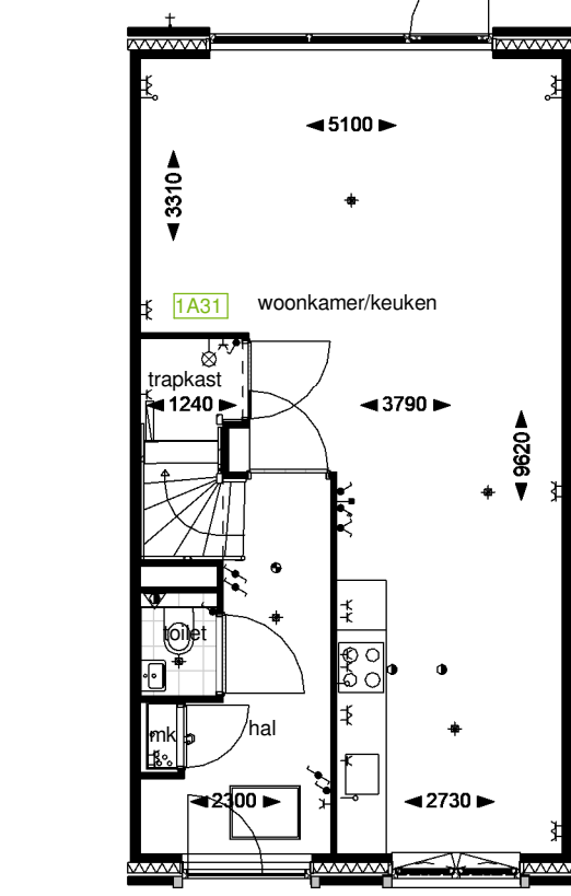
Optie C13.1: Principe trapkast bnr: 56 t/m 65, 79 t/m 88, 89 t/m 101
