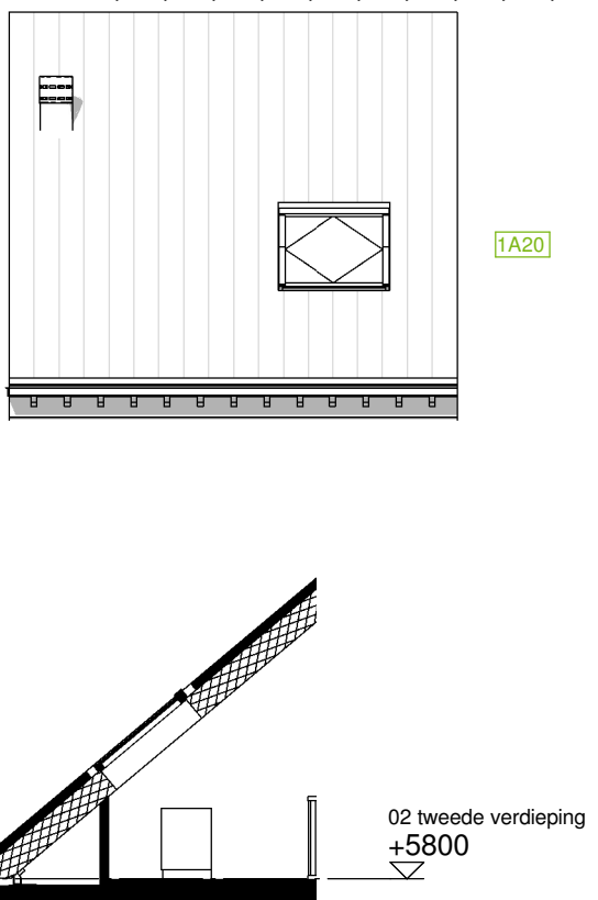
Optie C7.1: Principe dakraam voorgevel afmeting 1,34 x 1,40m bnr: 56, 58, 60, 61, 84, 86, 87, 92, 93, 97, 98
