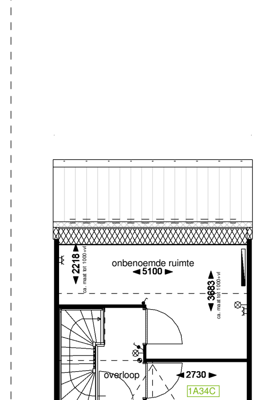
Optie C11.3: Principe zolderindeling bnr: 79, 80, 85, 88
