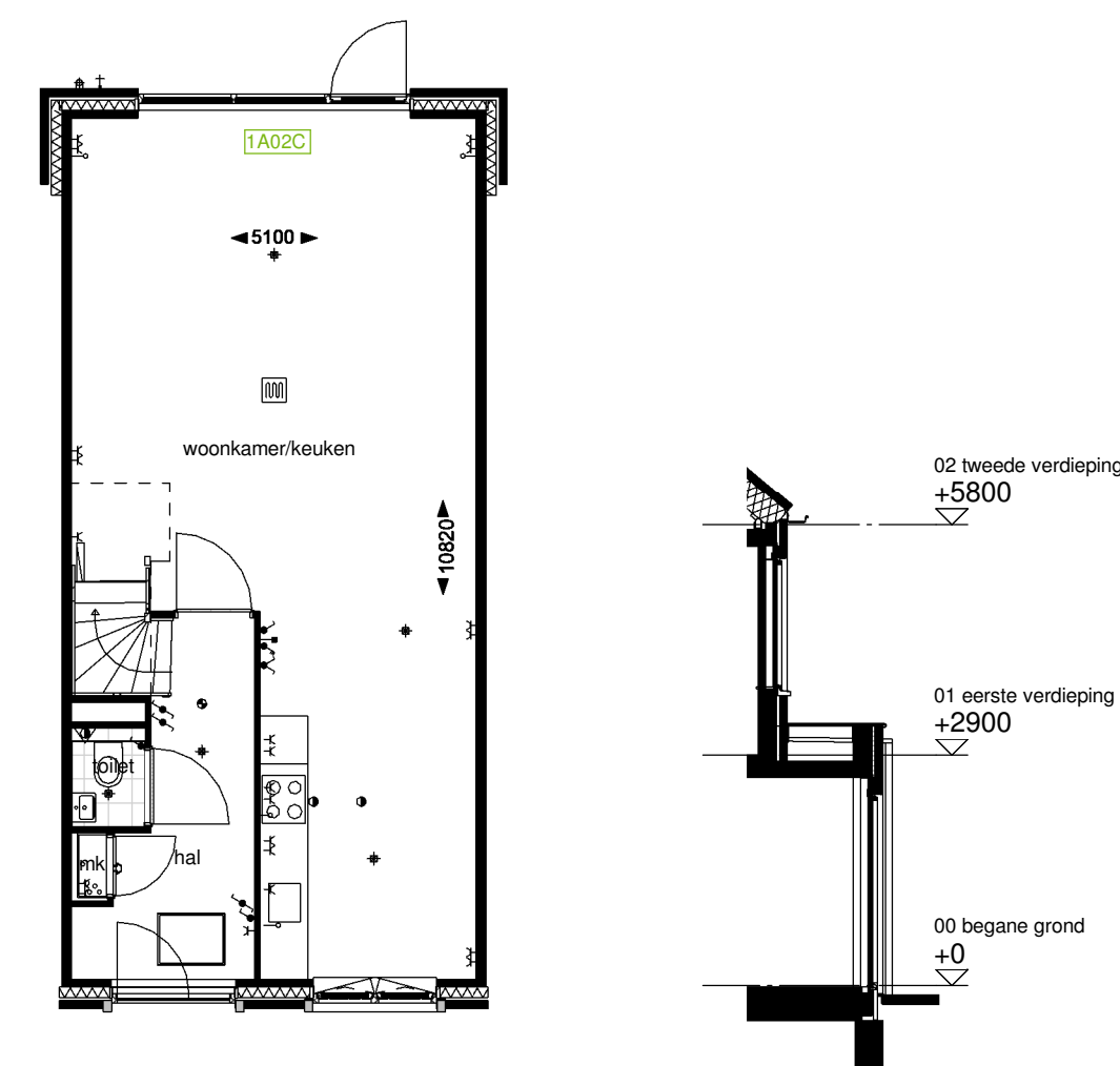
Optie C5.1: Principe dakkapel op de voorgevel bnr: 56, 58, 60, 61, 84, 96, 97, 92, 93, 97, 98
