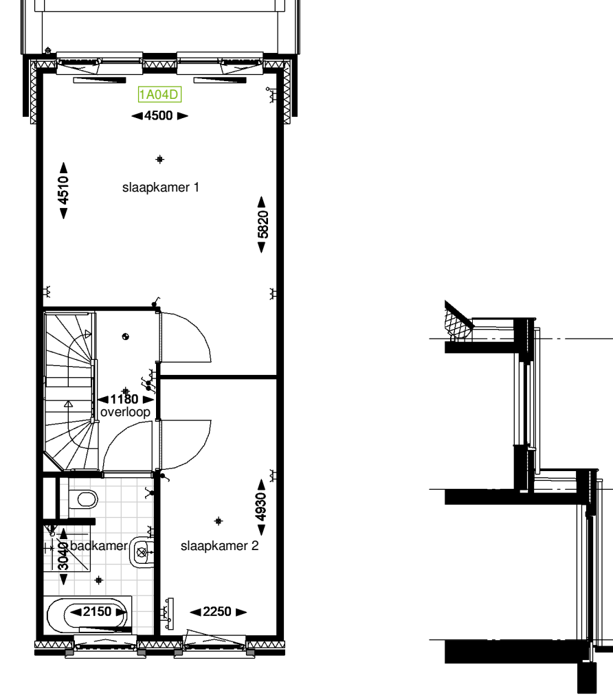
Optie D12.1: Principe grote pui met dubbele deur achtergevel bnr: 135 t/m 139
