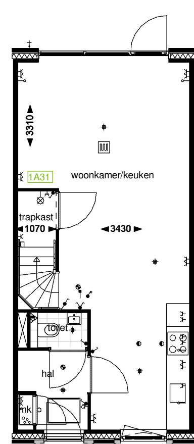
Optie D13.1: Principe trapkast bnr: 135 t/m 139
