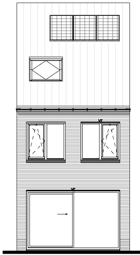
Optie D14.1: Principe schuifpui bnr: 135 t/m 139
