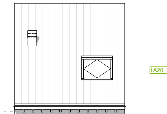
Optie D7.1: Principe dakraam voorgevel afmeting 1,34 x1,40m bnr: 137, 139
