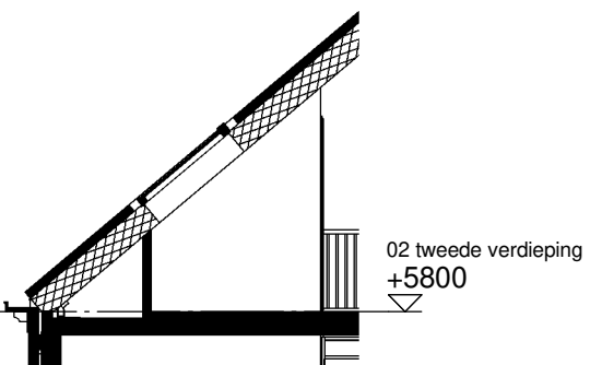
Optie D8.1: Principe dakraam achtergevel afmeting 1,34 x1,40m bnr: 135 t/m 139
