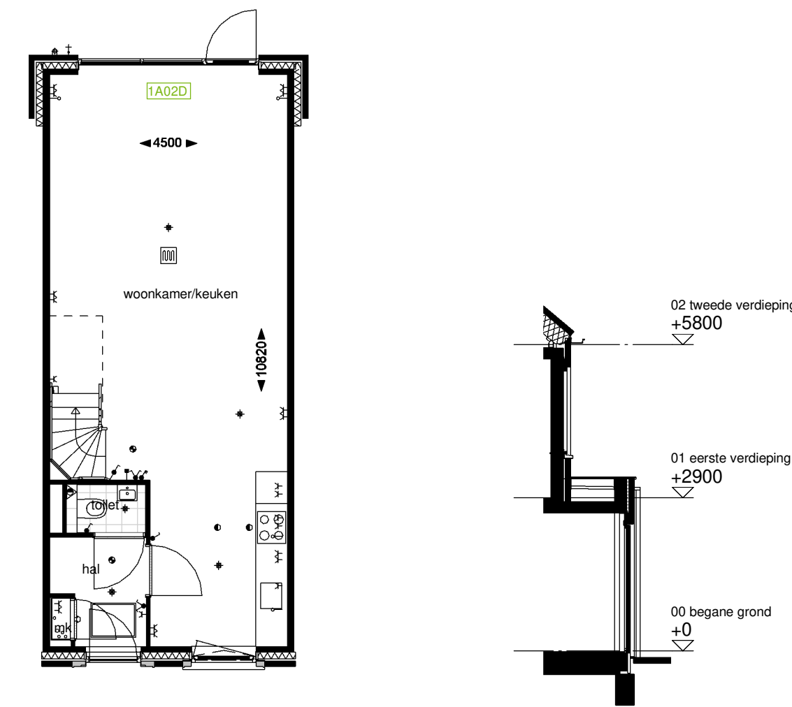
Optie D7.1: Principe dakraam voorgevel afmeting 1,34 x1,40m bnr: 137, 139
