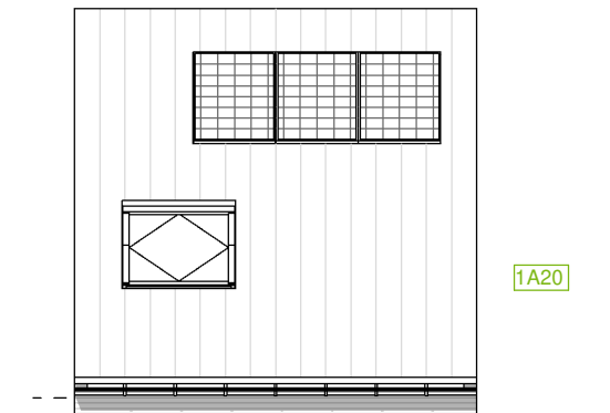
Optie D8.1: Principe dakraam achtergevel afmeting 1,34 x1,40m bnr: 135 t/m 139
