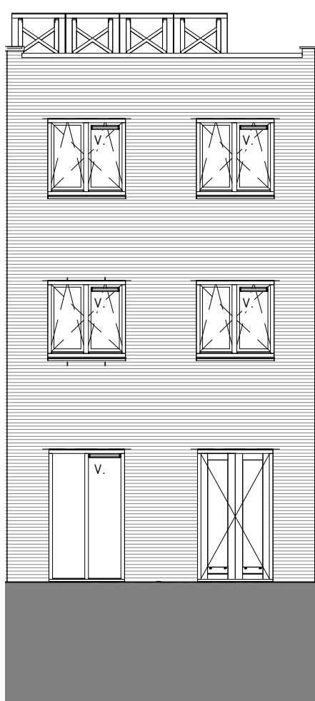
Achtergevel bwnr 22,25,31,34,36
