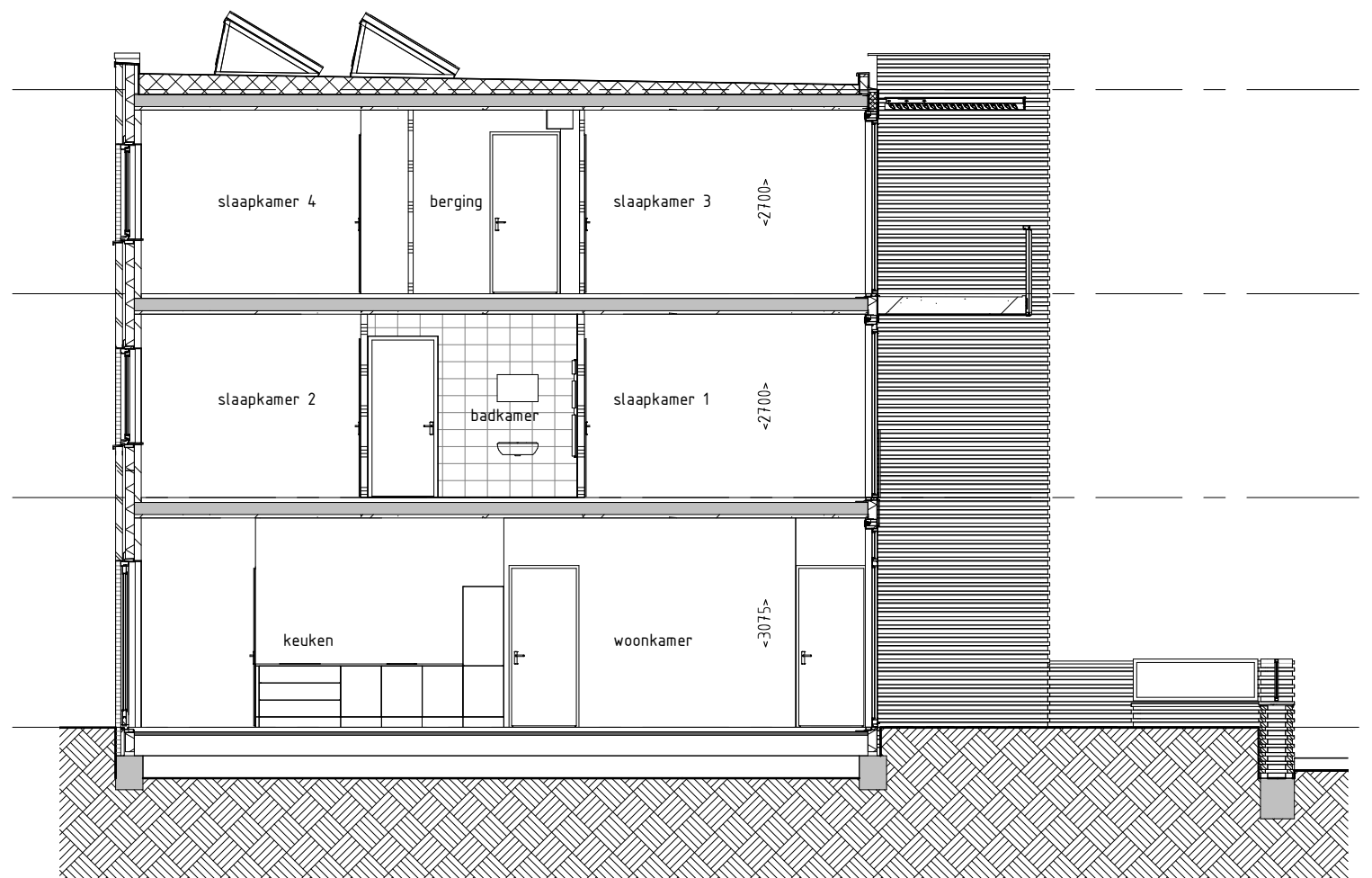
Doorsnede
