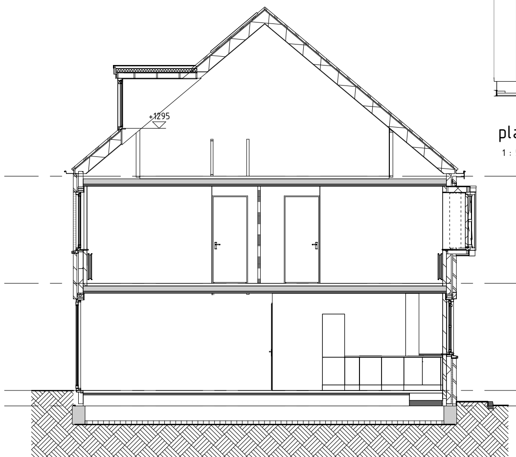
doorsnede
