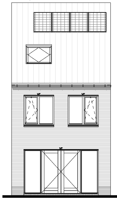
Optie C12.1: Principe grote pui met dubbele deuren achtergevel bnr: 112 t/m 117, 118 t/m 134
