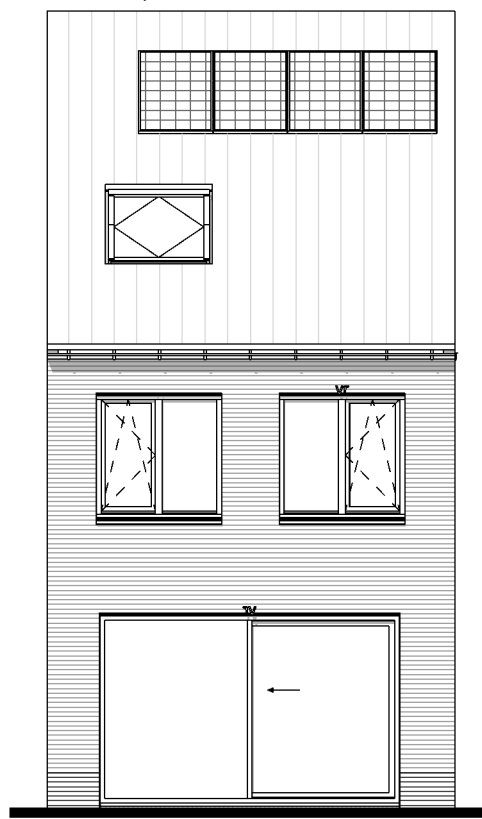
Optie C15.1: Principe schuipui bnr: 112 t/m 117, 118 t/m 134
