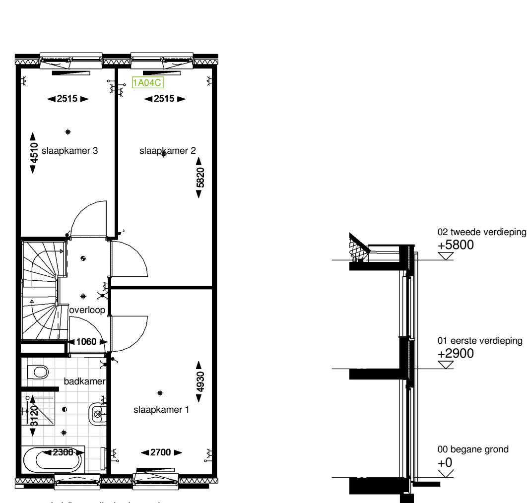
Optie C15.1: Principe schuipui bnr: 112 t/m 117, 118 t/m 134
