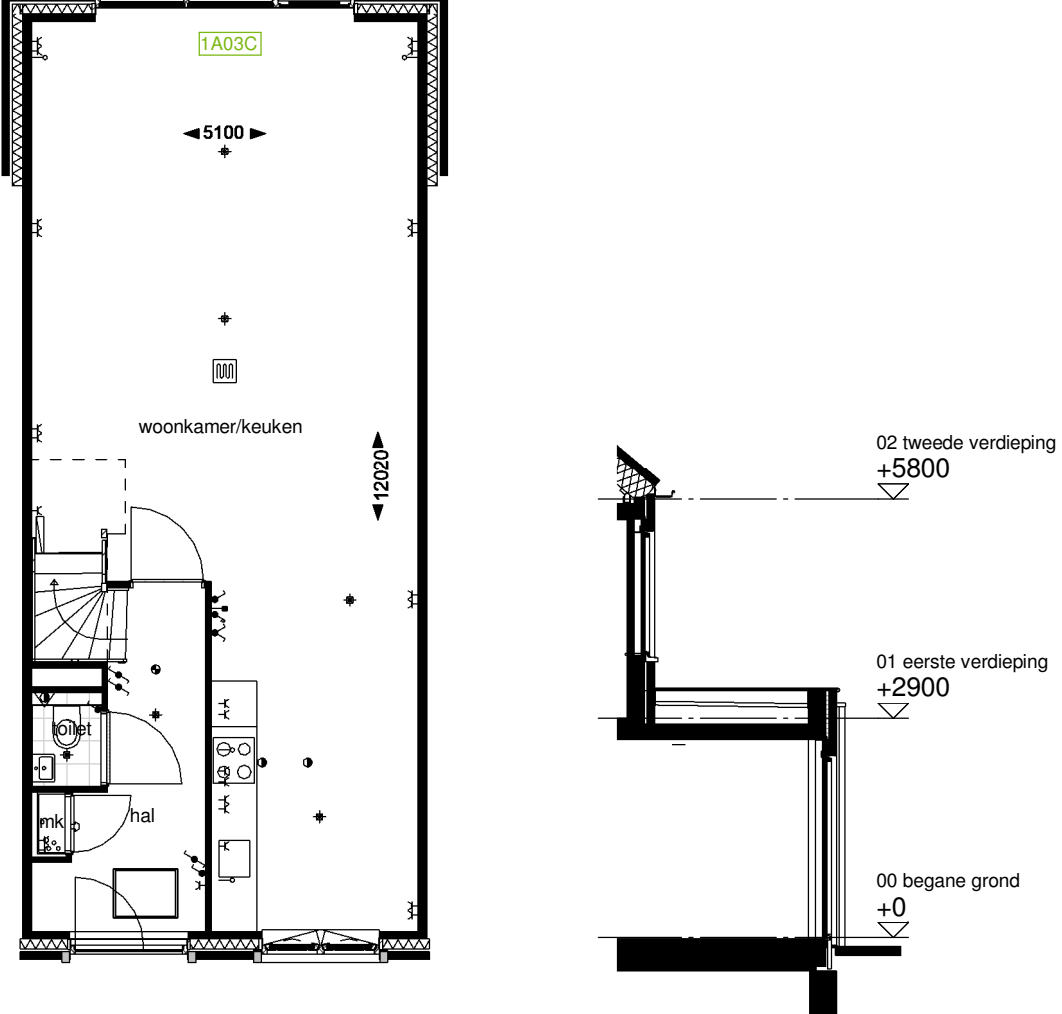
Optie C7.1: Principe dakraam voorgevel afmeting 1,34 x 1,40m bnr: 113, 115, 117, 123, 127, 129, 131
