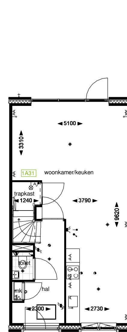
Optie C13.1: Principe trapkast bnr: 112 t/m 117, 118 t/m 134
