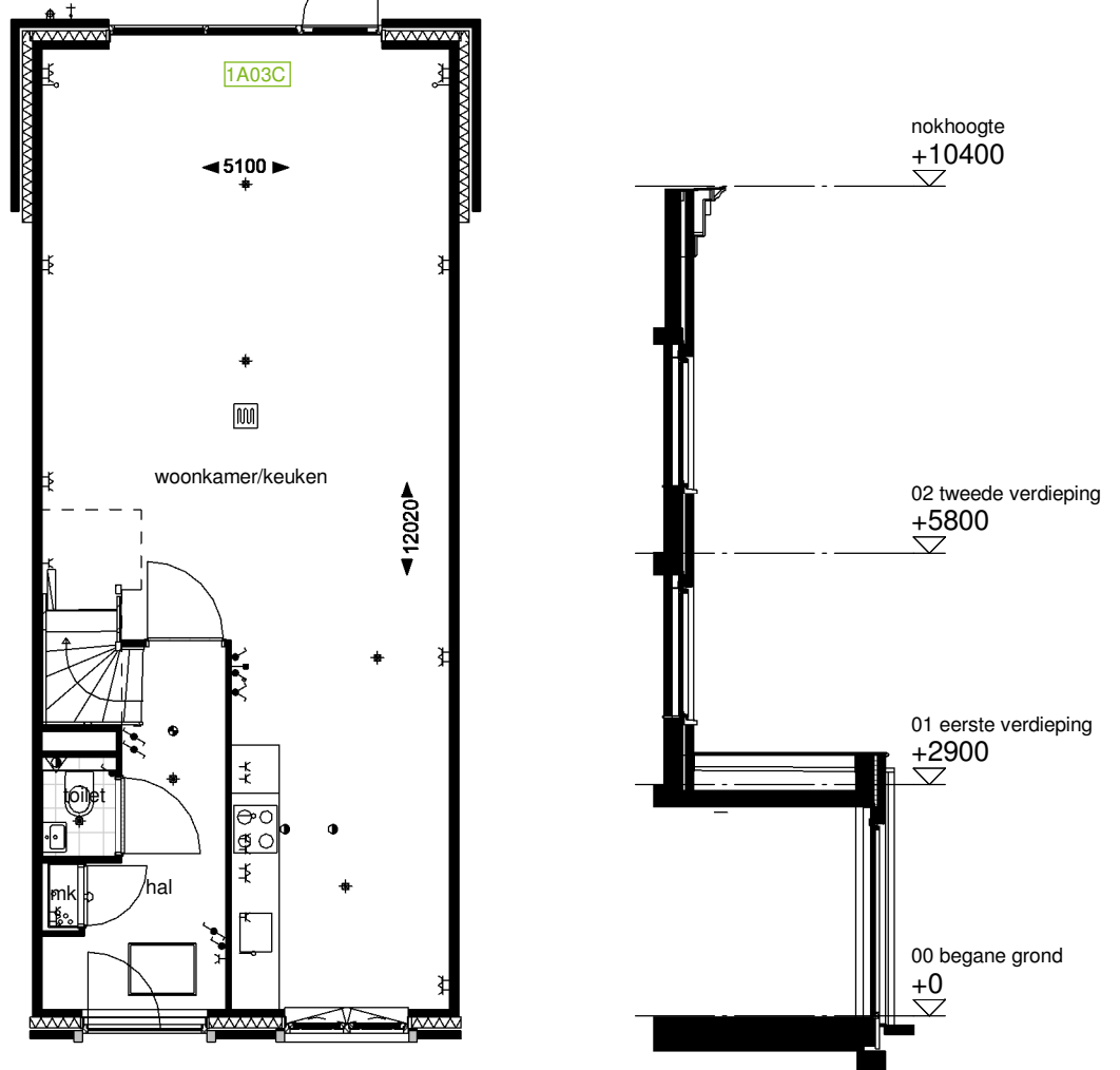
Optie C12.1: Principe grote pui met dubbele deuren achtergevel bnr: 112 t/m 117, 118 t/m 134
