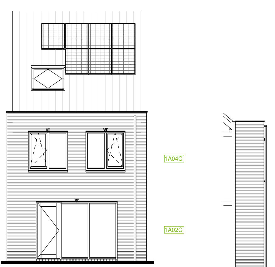
Optie C3.1: Principe uitbouw achterzijde woonkamer met ca. 1,2meter en de 1e verdieping ca. 1,2m bnr: 112 t/m 117, 119 t/m 133
