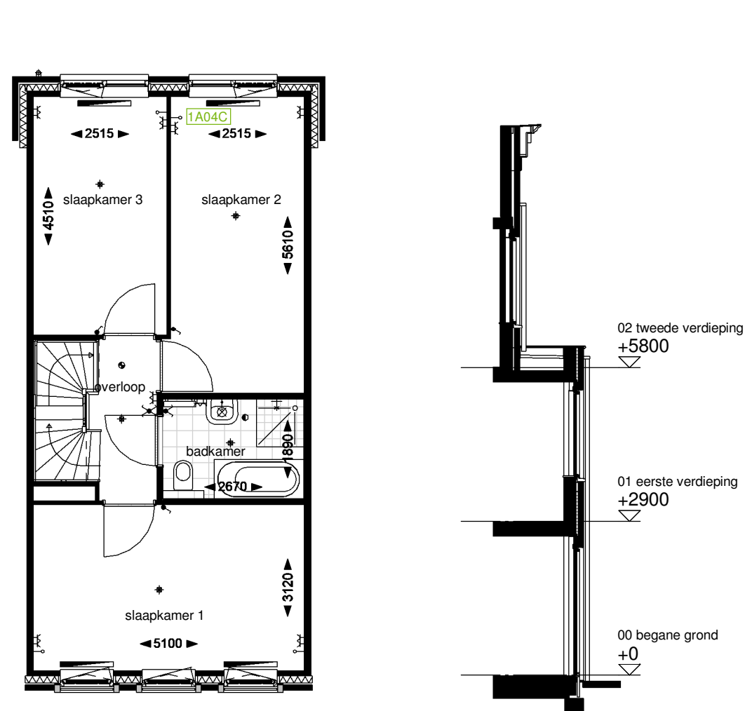
Optie C9.1: Principe indeling midden badkamer bnr: 113, 114, 127 t/m 131
