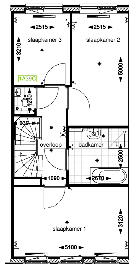
Optie C10.1: Principe indeling midden badkamer met apart toilet (alleen iem optie C3.1 / C3.2 en C13.1) bnr: 115 t/m 126 en 132 t/m 134
