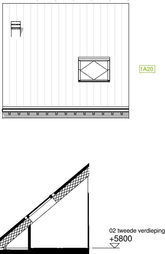
Optie C7.1: Principe dakraam voorgevel afmeting 1,34 x 1,40m bnr: 113, 115, 117, 123, 127, 129, 131
