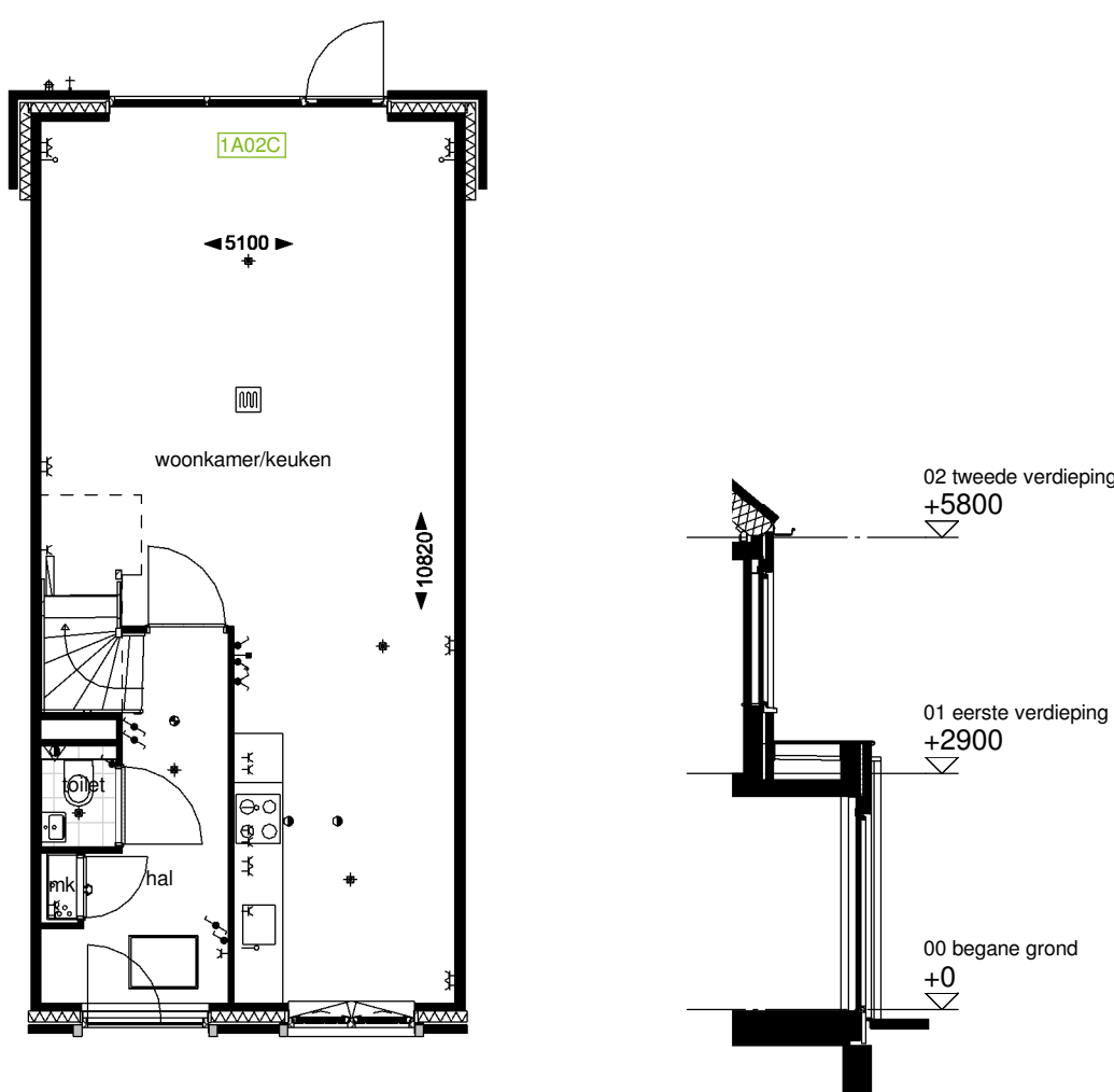
Optie C5.1: Principe dakkapel op de voorgevel bnr: 113, 115, 117, 123, 127, 129, 131
