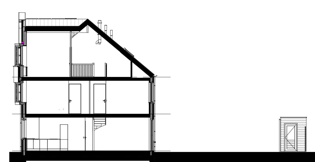
Doorsnede type A3 1 : 150
