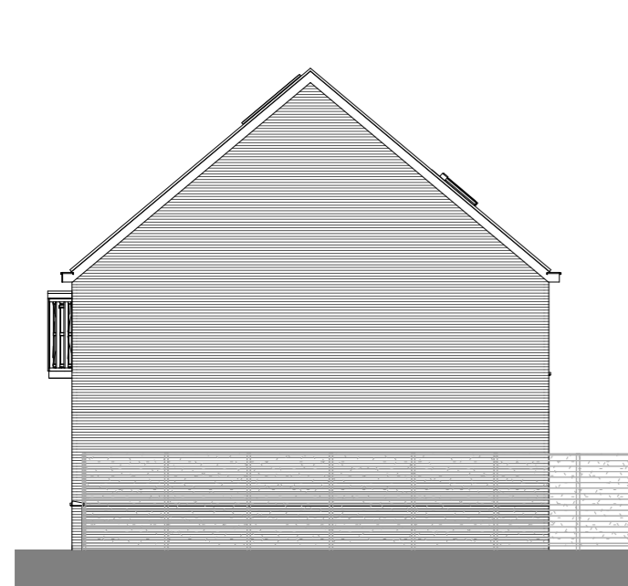
zijgevel rechts bwnr. 52 type A1H gespiegeld 1 : 150
