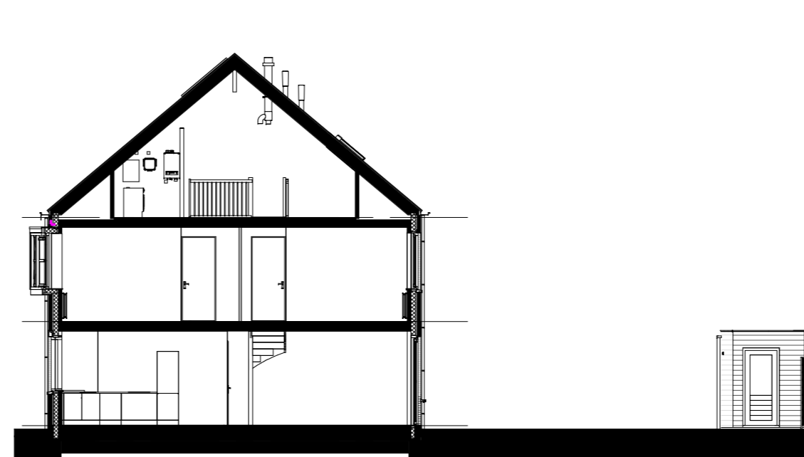
Doorsnede type A1 1 : 150
