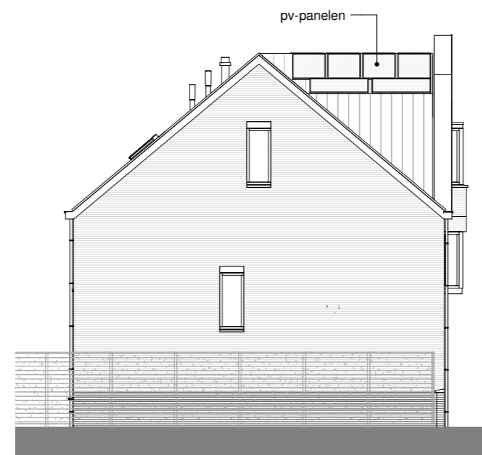
zijgevel links bwnr. 41 type A3H gespiegeld 1 : 150
