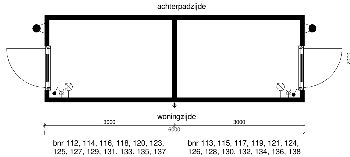
plattegrond
